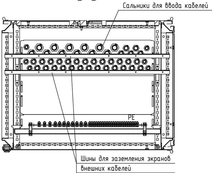
Б-Б
